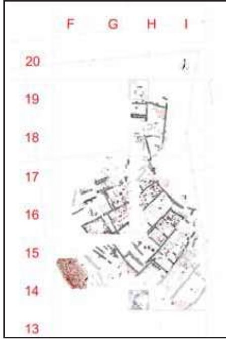
Çizim 3: VI No.lu Alan ,Yassitepe Höyüğü ETÇ mimarisi.
